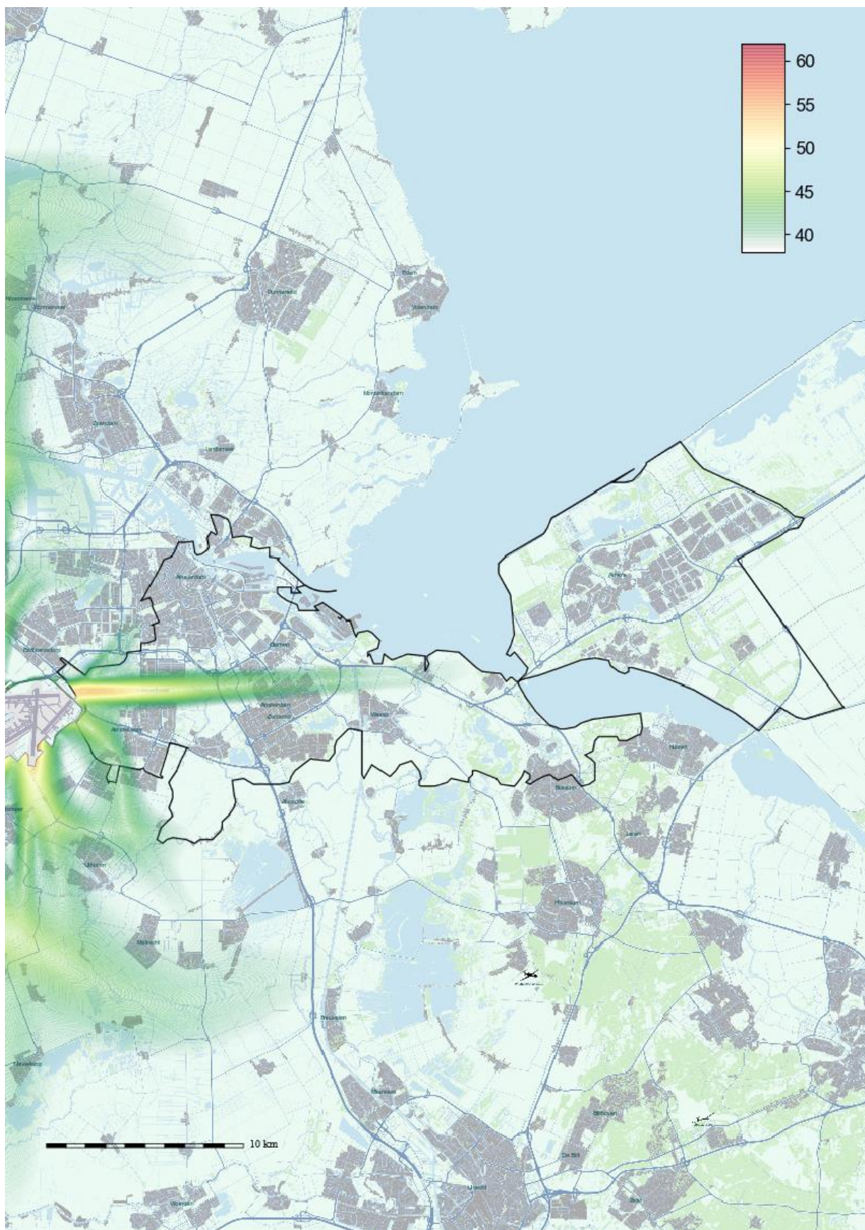
Cluster Buitenveldertbaan, kaart 4: Geluidbelasting gedurende de nacht (23.00 – 07.00) in Lnight dB(A).
