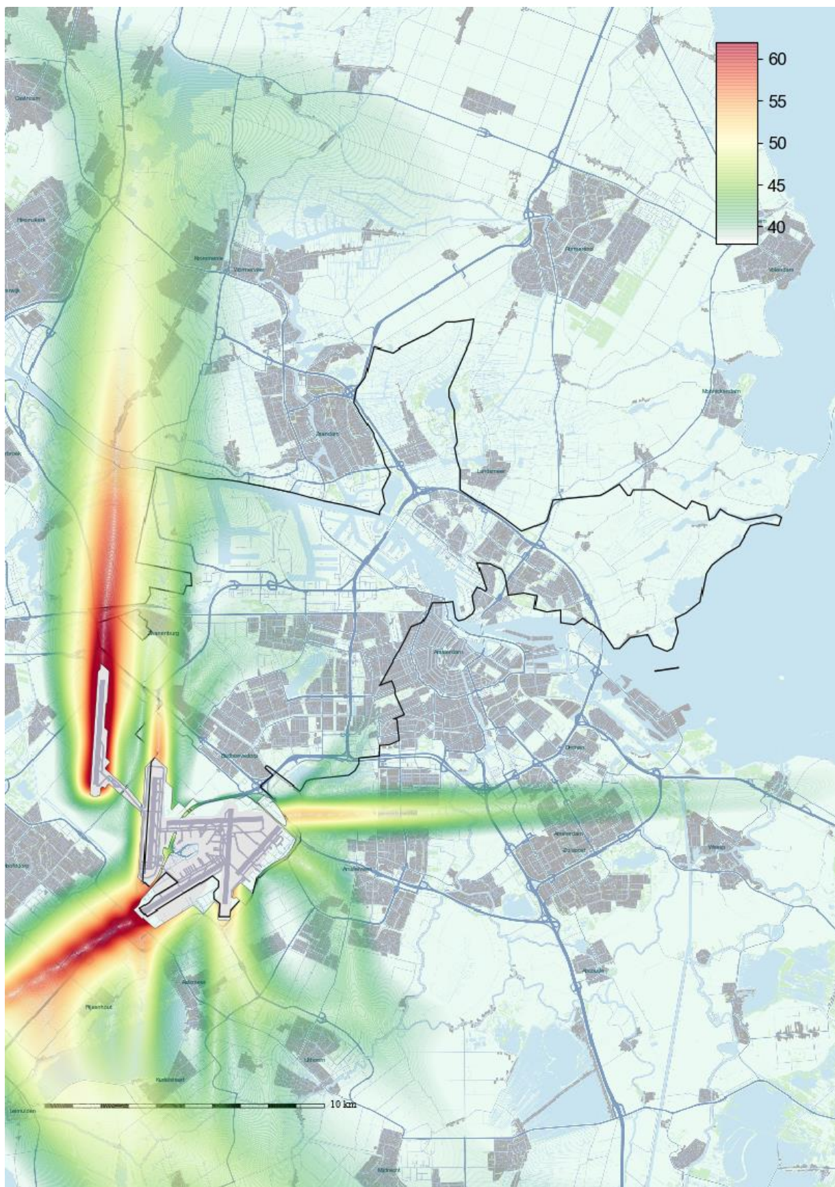
Cluster Zwanenburgbaan, kaart 10: Geluidbelasting gedurende de nacht (23.00 – 07.00) in Lnight dB(A).
