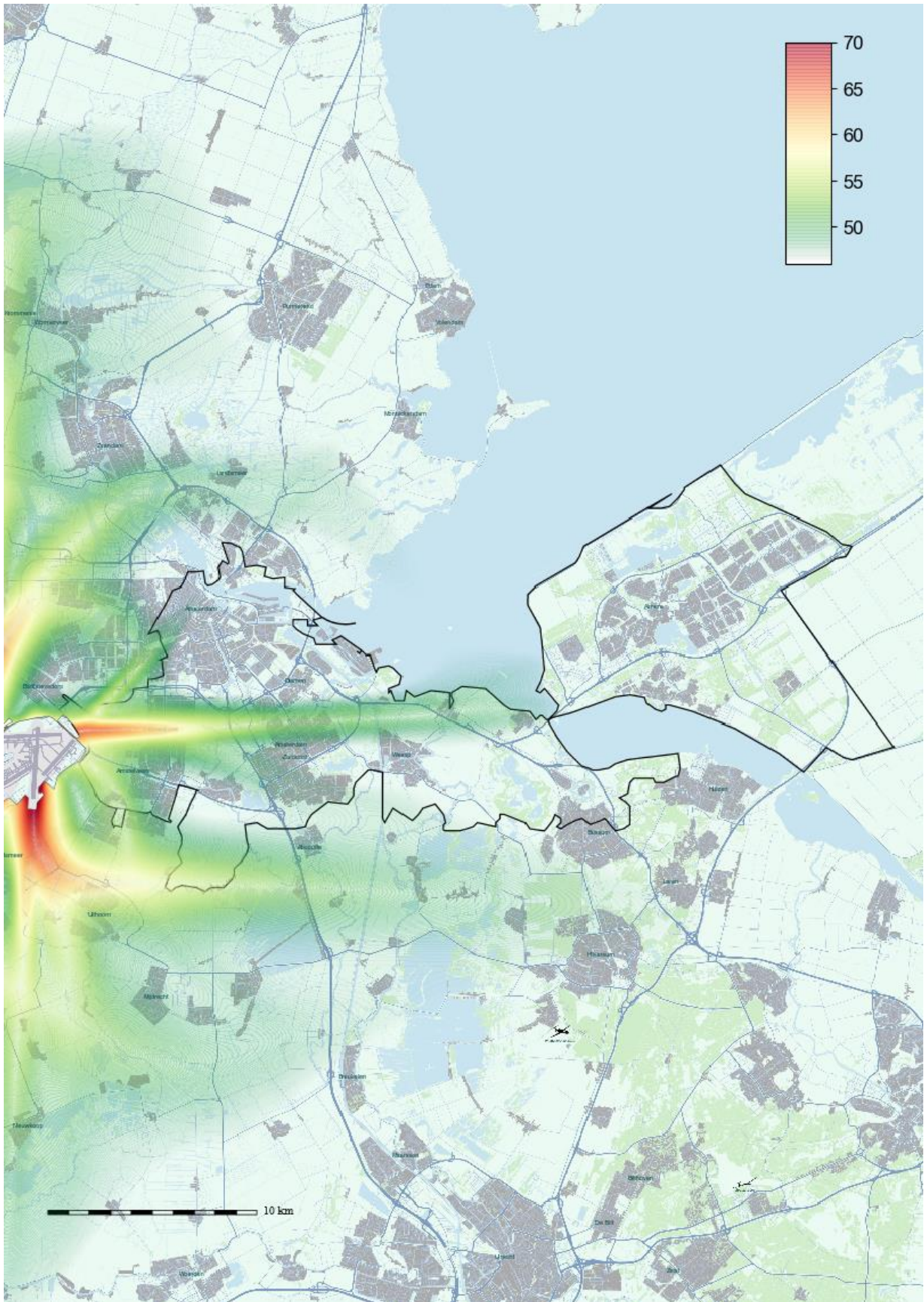
Cluster Buitenveldertbaan, kaart 3: Geluidbelasting in gebruiksjaar 2020 over het etmaal in Lden dB(A).
