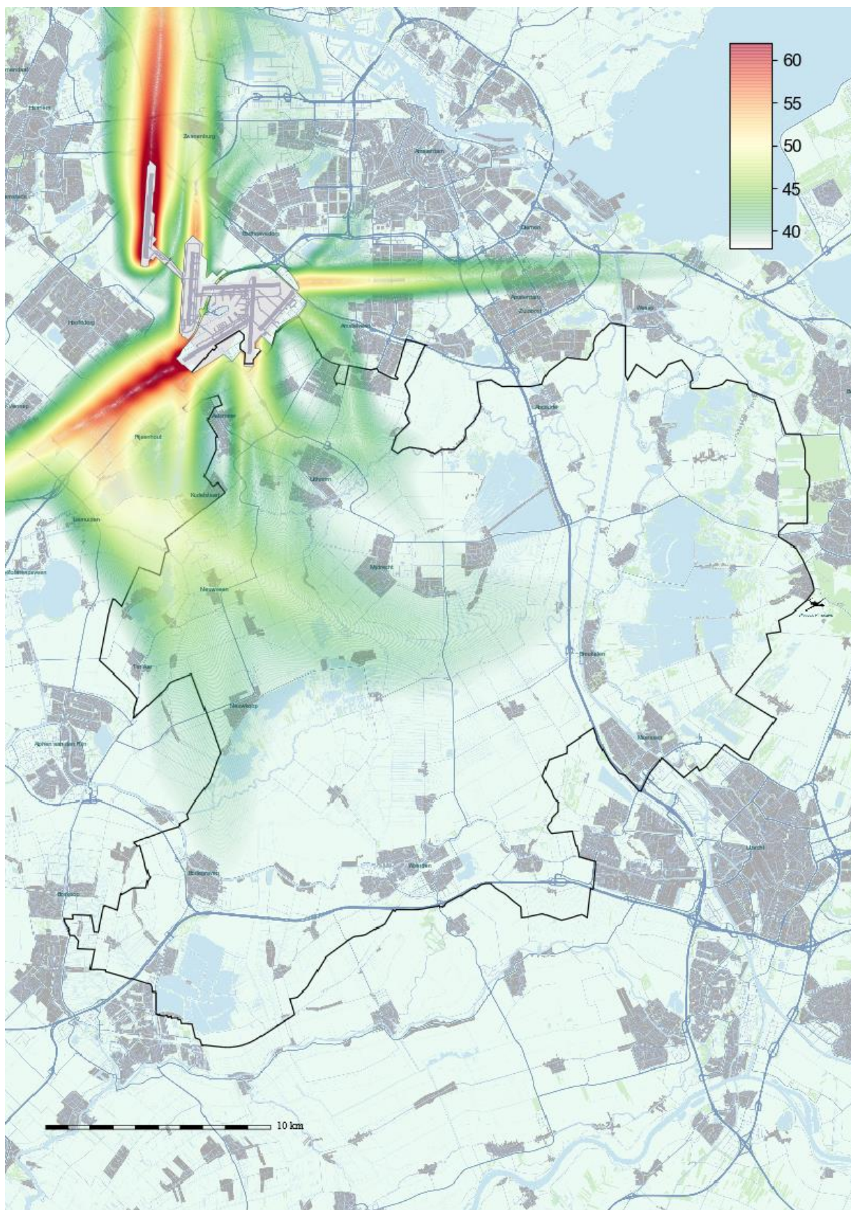
Cluster Aalsmeerbaan, kaart 2: Geluidbelasting gedurende de nacht (23.00 – 07.00) in Lnight dB(A).
