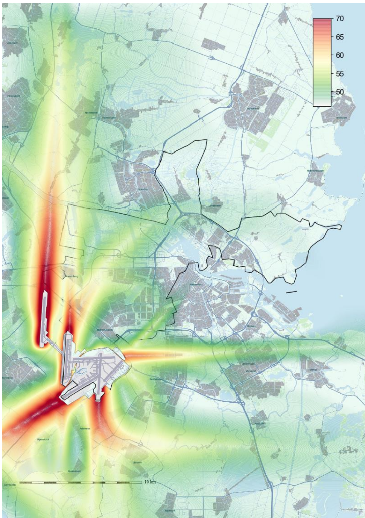
Cluster Zwanenburgbaan, kaart 9: Geluidbelasting in gebruikjaar 2020 over het etmaal in Lden dB(A).
