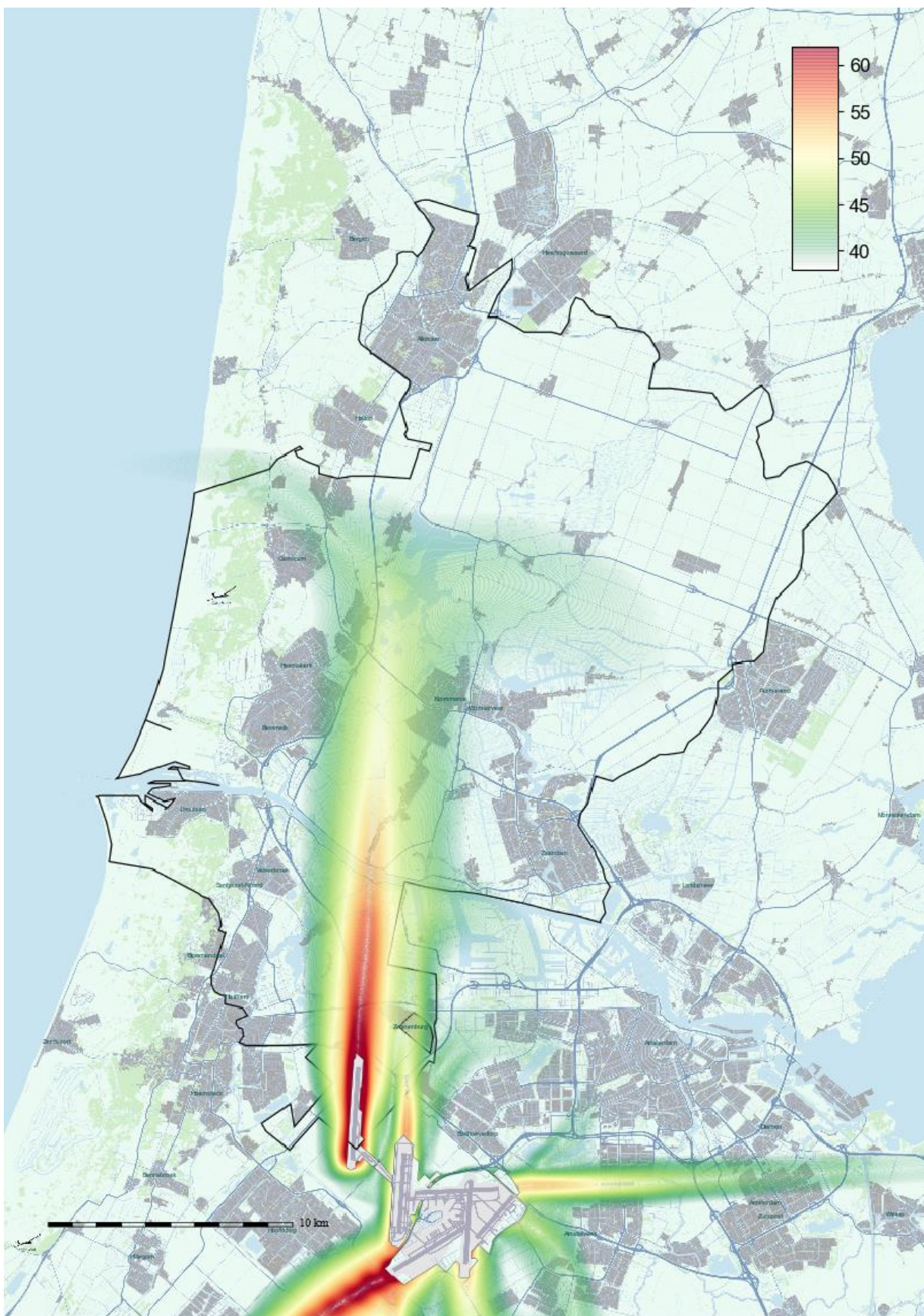
Cluster Polderbaan, kaart 8: Geluidbelasting gedurende de nacht (23.00 – 07.00) in Lnight dB(A).
