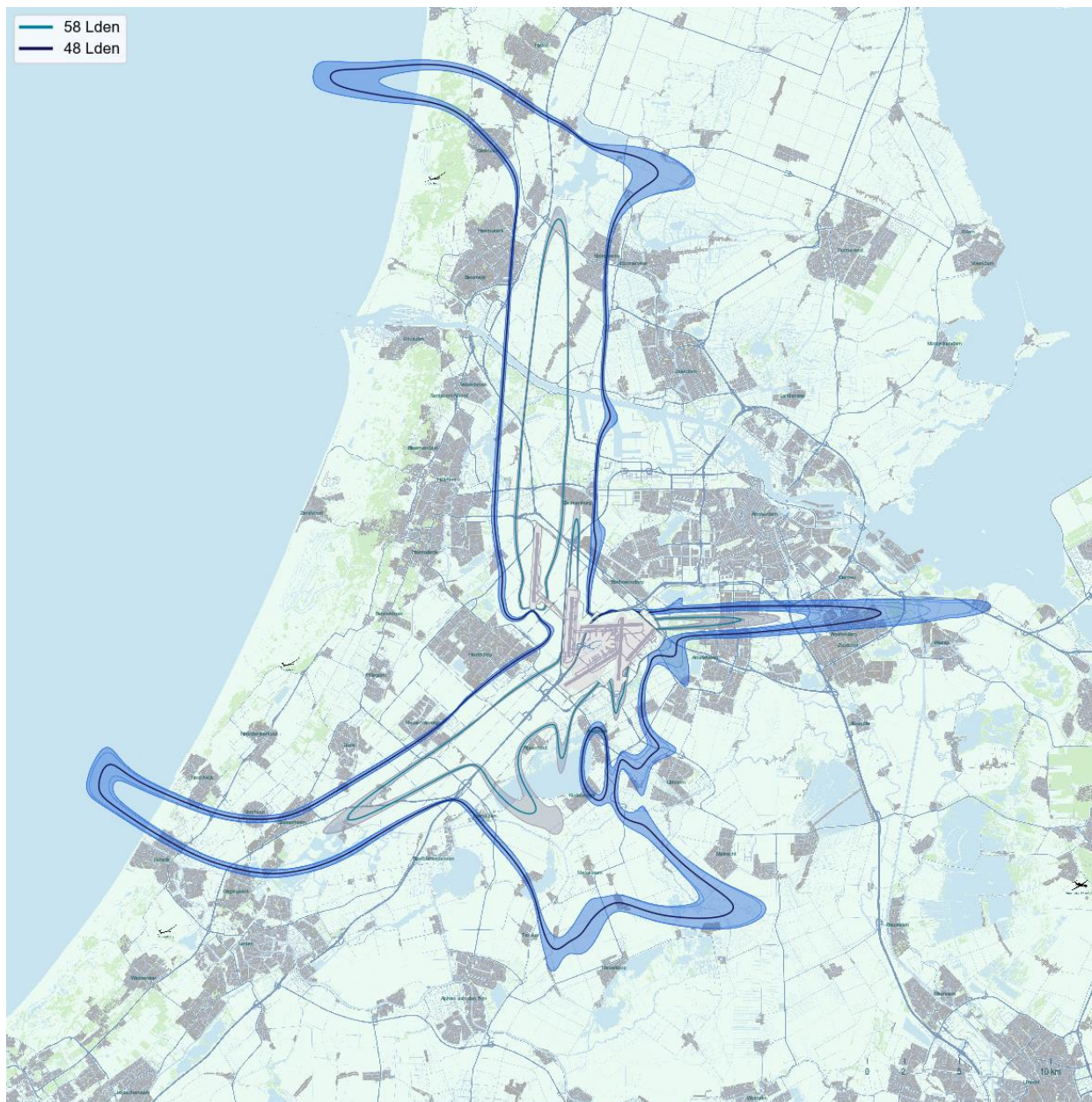
Figuur 5.2: Verwachte jaargemiddelde geluidbelasting over de nachtperiode L_{\text{night}} voor gebruikjaar 2020, met spreiding als gevolg van weersvariaties.
