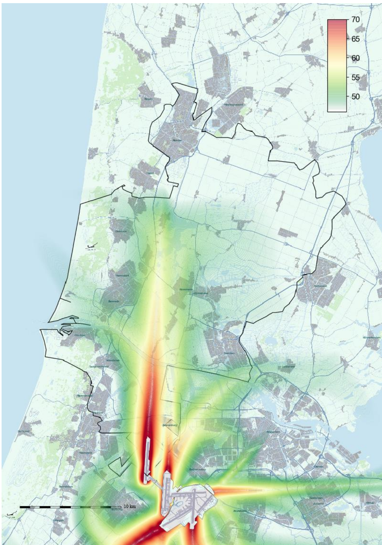
Cluster Polderbaan, kaart 7: Geluidbelasting in gebruikjaar 2020 over het etmaal in Lden dB(A).
