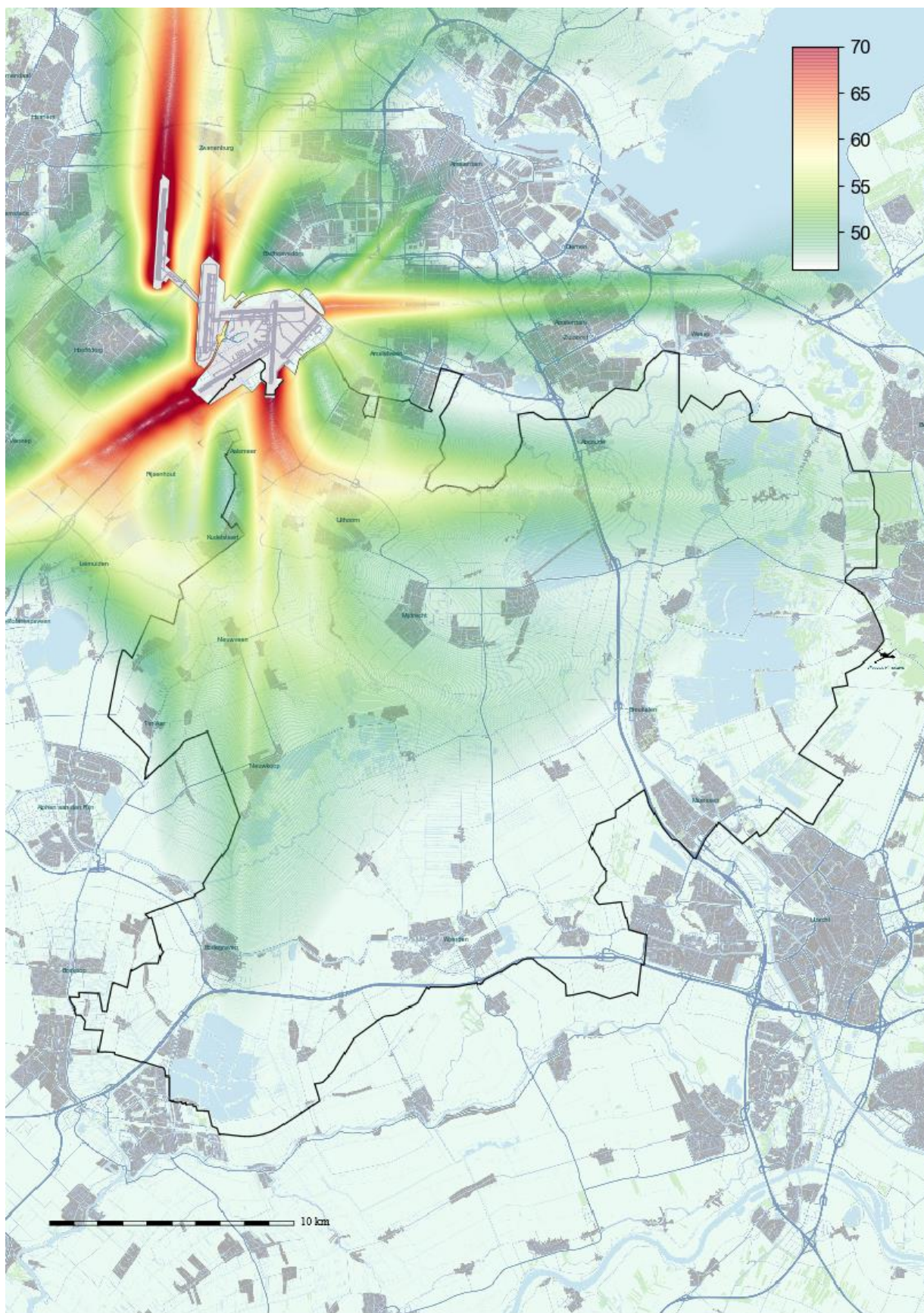
Cluster Aalsmeerbaan, kaart 1: Geluidbelasting in gebruiksjaar 2020 over het etmaal in Lden dB(A).
