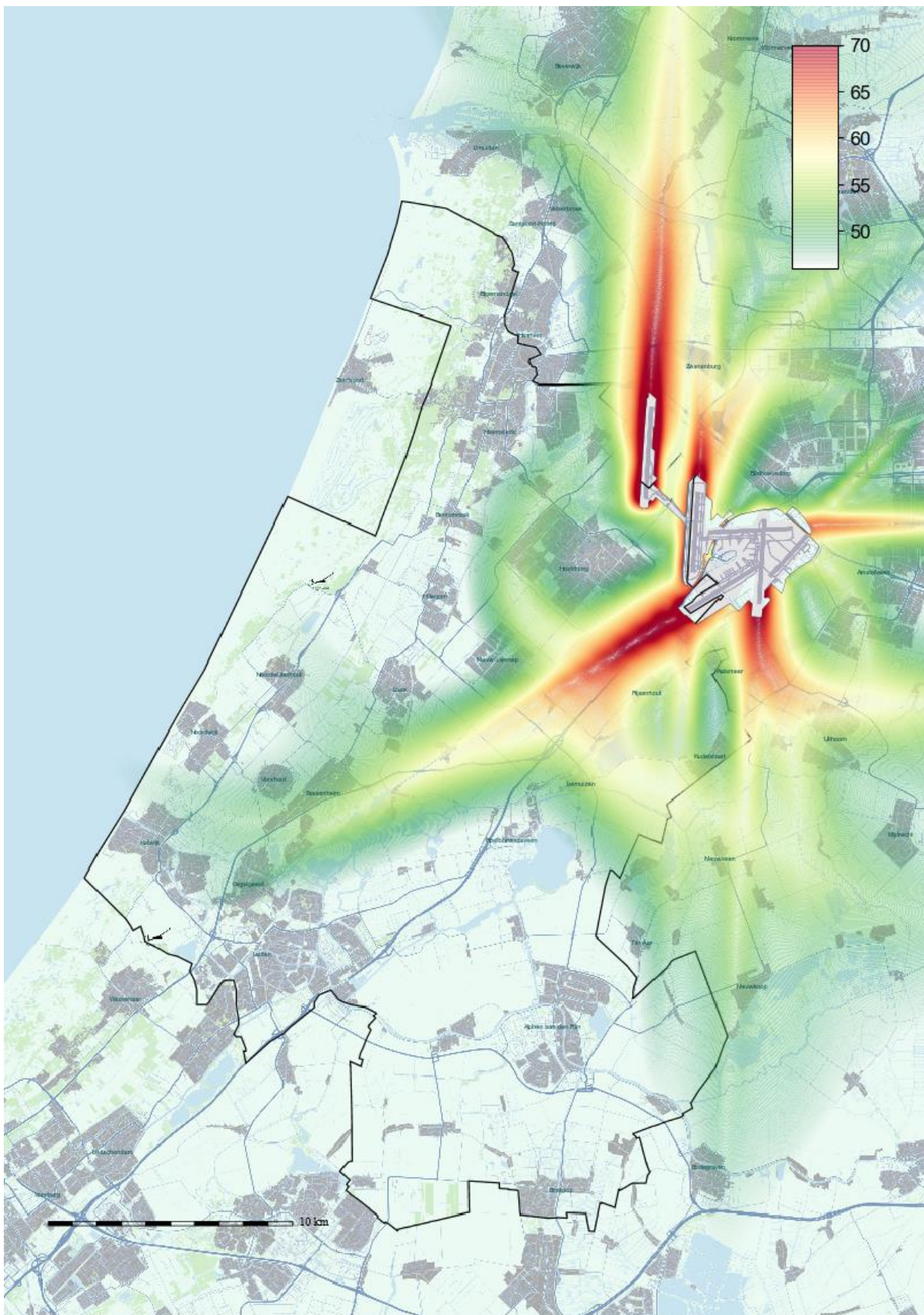
Cluster Kaagbaan, kaart 5: Geluidbelasting in gebruikjaar 2020 over het etmaal in Lden dB(A).
